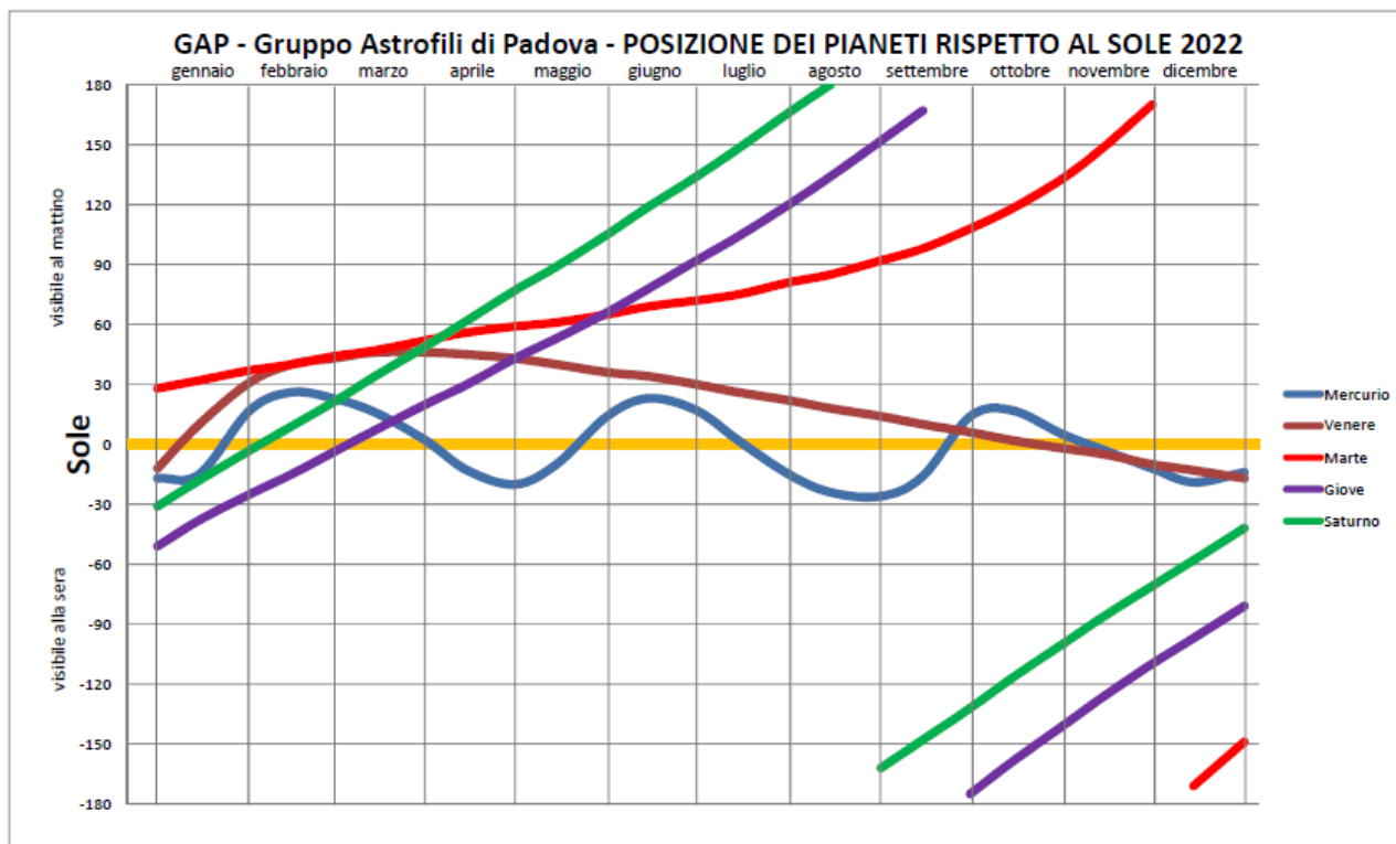
Figura 1. Posizione apparente dei pianeti rispetto al Sole nel 2022.
