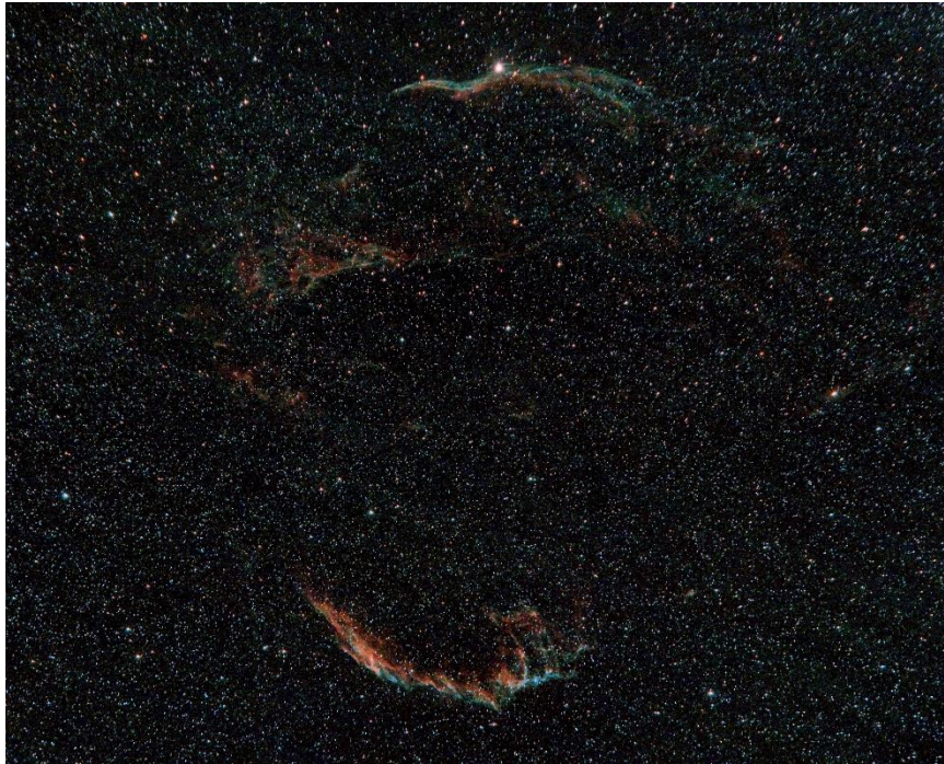
Figura 4. Nebulosa Velo
