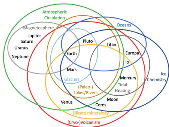
Figura 3. Diagramma di Wenn che mostra come pianeti e satelliti condividano moltissime caratteristiche, indipendentemente dal tipo di orbita che seguono.
